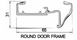
ROUND DOOR FRAME
